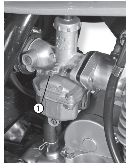
Рис. 20. Карбюратор
