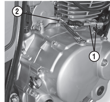
Рис. 16. Регулировка сцепления
