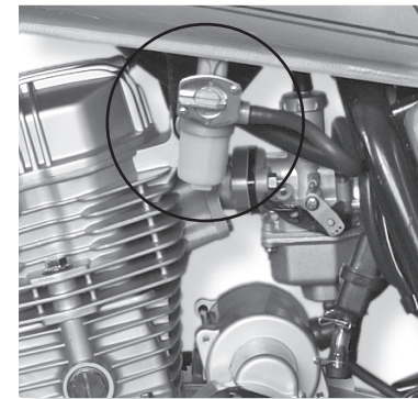
Рис. 11 Топливный кран
