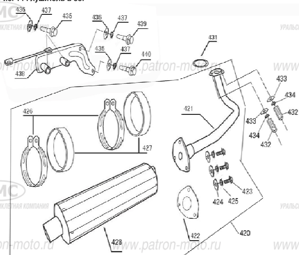
Рис. 14 Глушитель в сб.
