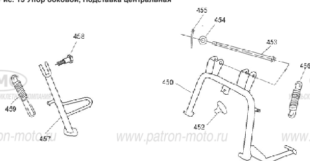
Рис. 15 Упор боковой, Подставка центральная
