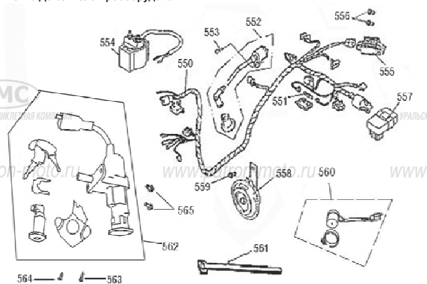
Рис. 19 Детали электрооборудования
