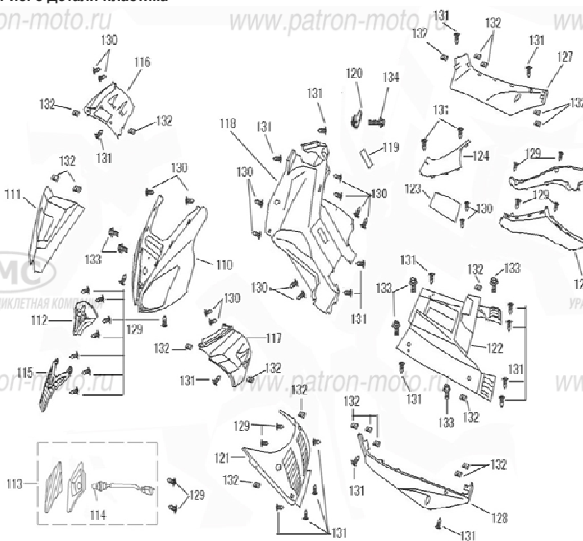
Рис. 5 Детали пластика
