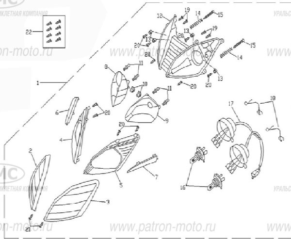
Рис. 1 ФАРА В СБ.
