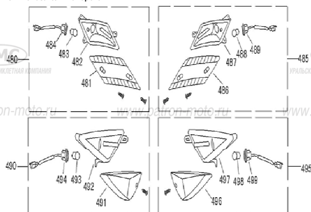
Рис. 17 Указатели поворотов
