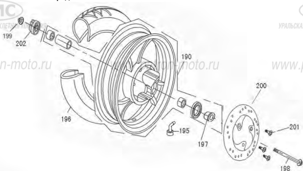
Рис. 7 Колесо переднее в сб.
