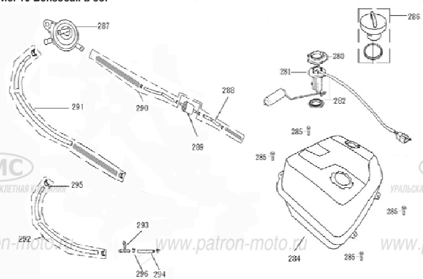
Рис. 10 Бензобак в сб.
