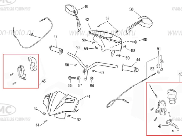
Рис. 3 Руль в сб.
