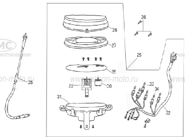
Рис. 2 КОМБИНАЦИЯ ПРИБОРОВ
