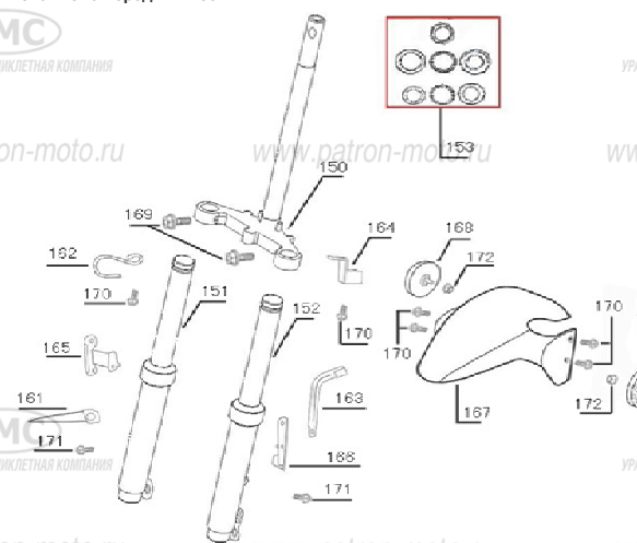
Рис. 6 Вилка передняя в сб.
