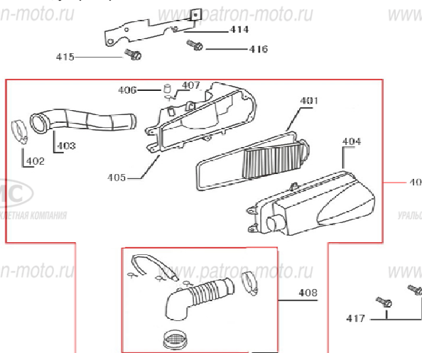
Рис. 13 Воздухофильтр
