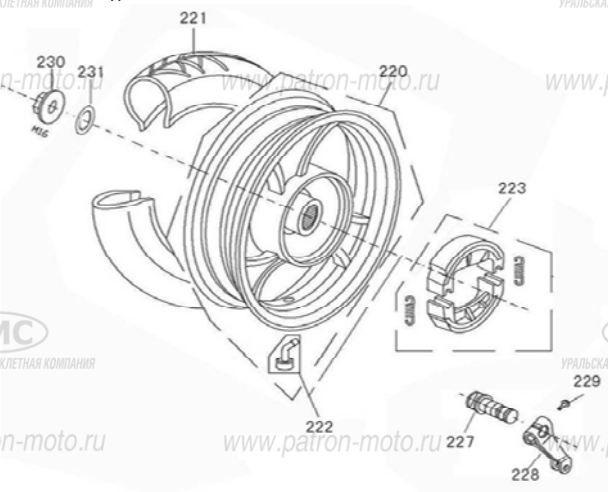
Рис. 8 Колесо заднее в сб.
