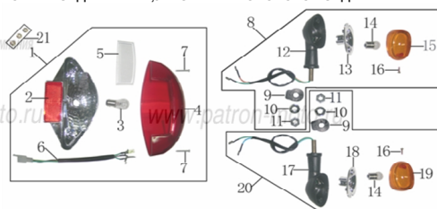
Рис. 12 ФОНАРЬ ЗАДНИЙ В СБ., УКАЗАТЕЛИ ПОВОРОТОВ ЗАДНИЕ
