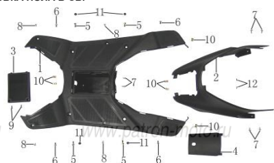
Рис. 9 ОБЛИЦОВКА ПОЛА В СБ.
