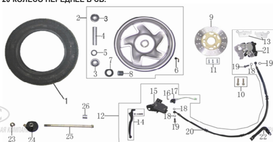
Рис. 20 КОЛЕСО ПЕРЕДНЕЕ В СБ.
