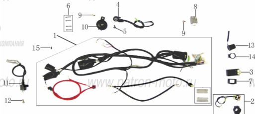
Рис. 16 ДЕТАЛИ ЭЛЕКТРОБОРУДОВАНИЯ
