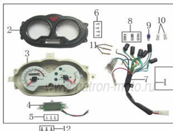
Рис. 2 КОМБИНАЦИЯ ПРИБОРОВ В СБ.
