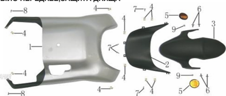
Рис. 10 КРЫЛО ПЕРЕДНЕЕ, ЗАЩИТА ДНИЩА
