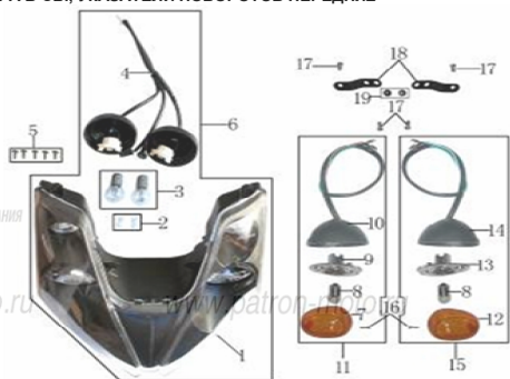
Рис. 4 ФАРА В СБ., УКАЗАТЕЛИ ПОВОРОТОВ ПЕРЕДНИЕ
