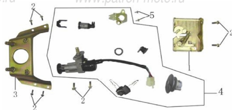
Рис. 13 КОМПЛЕКТ ЗАМКОВ
