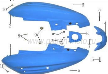
Рис. 8 ОБТЕКАТЕЛИ СЕДЛА
