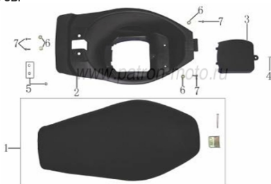
Рис. 8 ОБТЕКАТЕЛИ СЕДЛА
