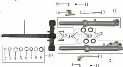
Рис. 19 ВИЛКА ПЕРЕДНЯЯ В СБ.
